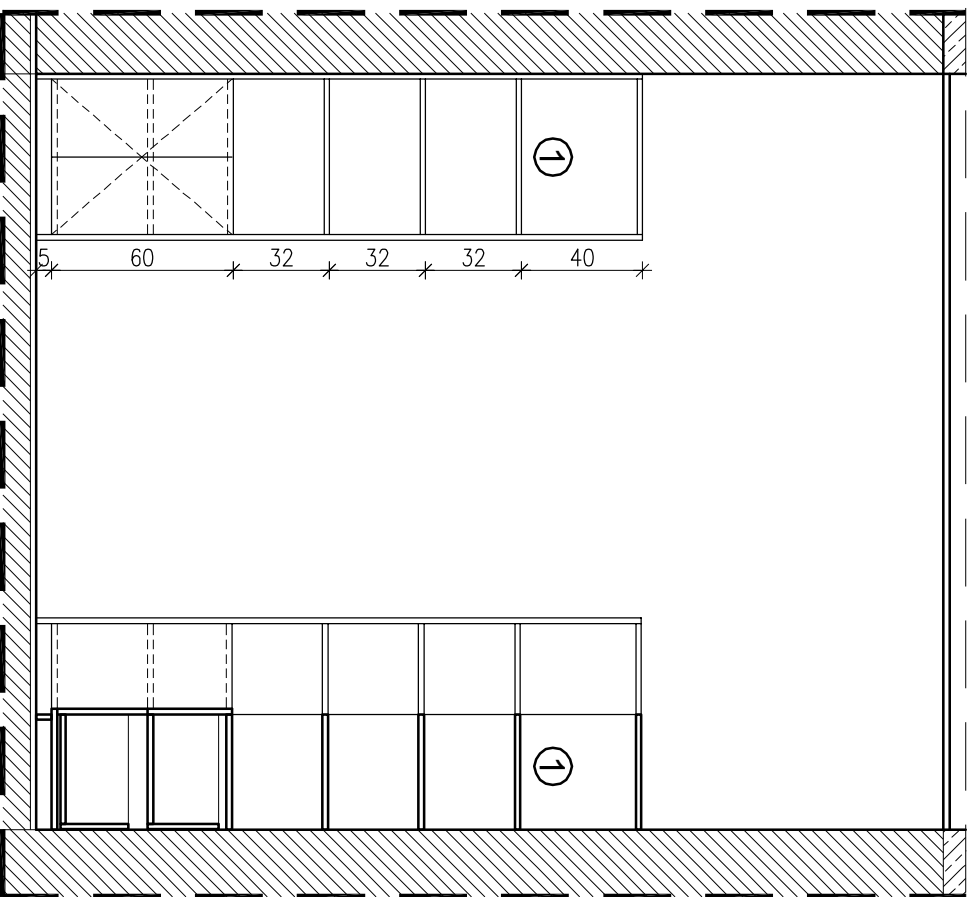
PRZEKRÓJ CC
