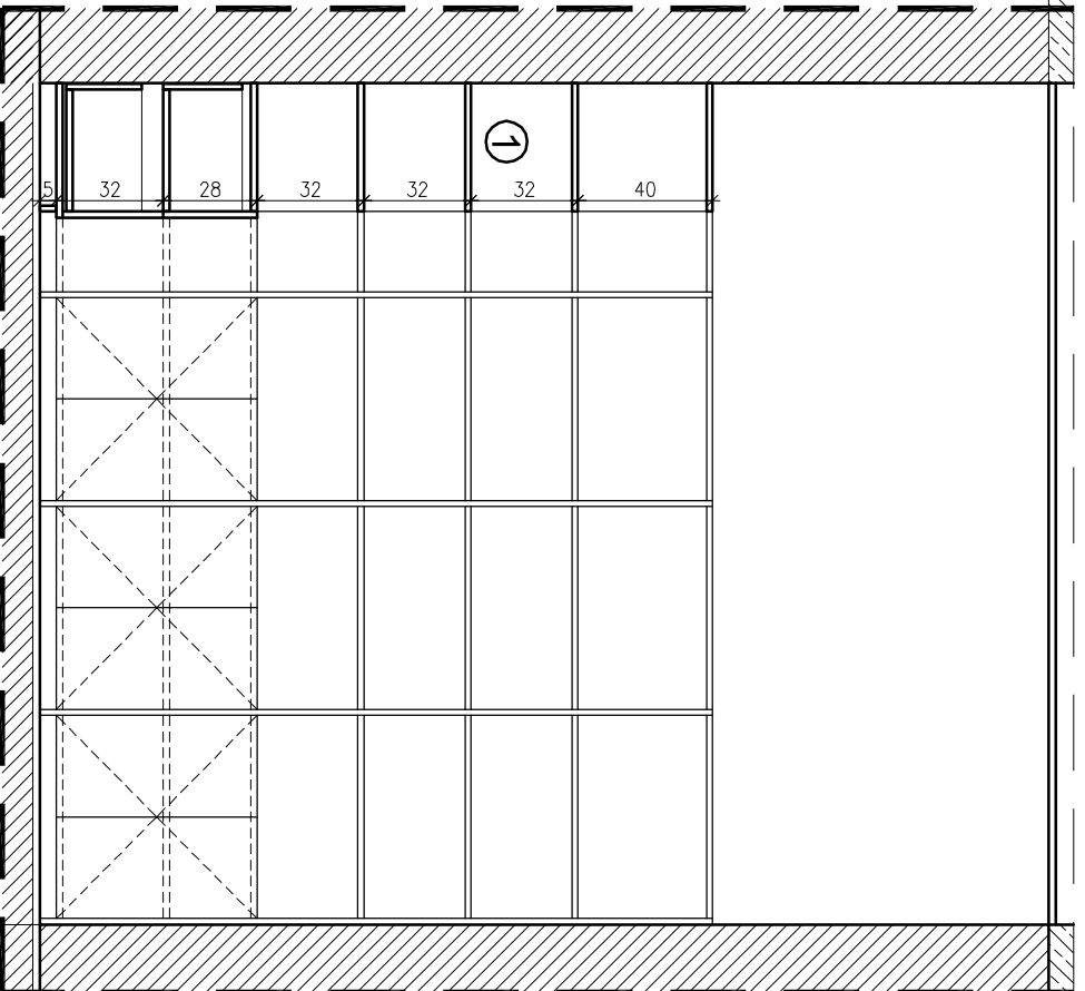
PRZEKRÓJ DD
